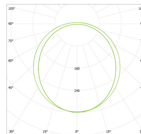
37W 4000K 1175x98mm
